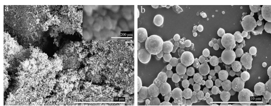
图 4 原始 \text{TiO}_2 (a) 和 PMMA-co-MAA/ \text{TiO}_2 复合粒子 (b) 的 SEM 图像 [9]
