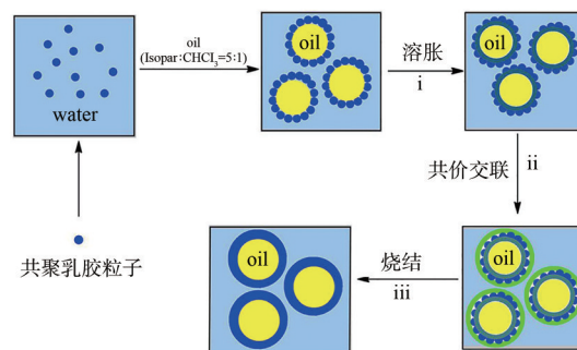
图 11 微胶囊制备方法示意图 [37]
