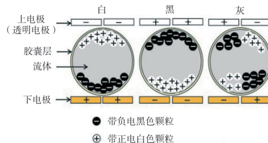
图1 电泳电子纸显示结构及工作原理 [2]
