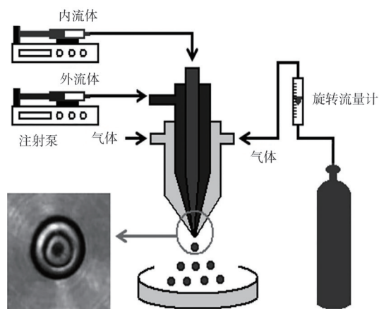
图12 用于EPD微胶囊制备的同轴喷射装置 [39]
