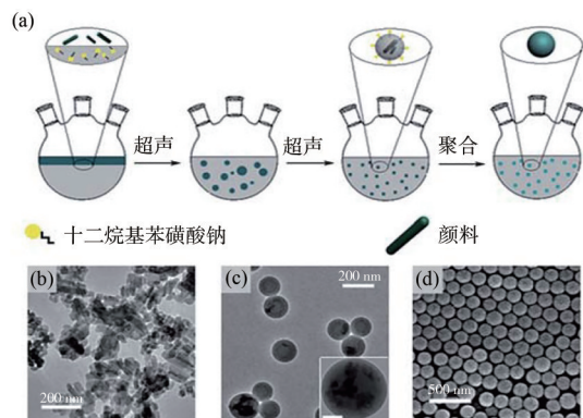
图6 (a)油墨颗粒的合成过程;(b)纯绿色颜料的SEM图像;(c)绿色油墨颗粒的SEM图像;(d)低倍下绿色油墨颗粒的SEM图像 [17] 。
