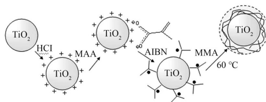
图2 PMMA 包覆 \text{TiO}_2 纳米粒子的示意图 [5]
