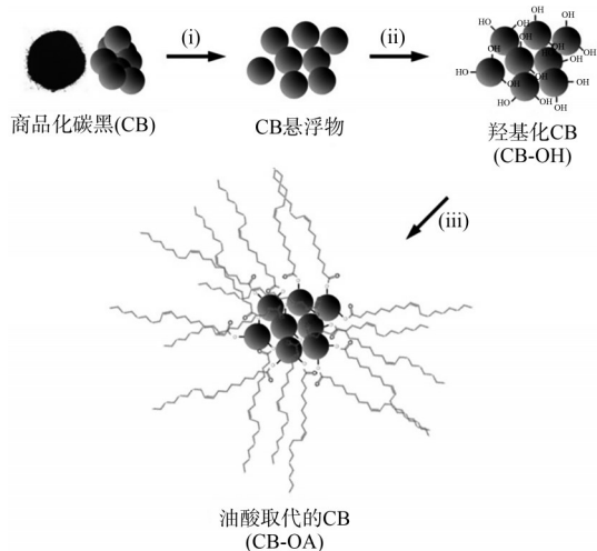
图9 碳黑粒子表面的油酸改性 [19]
