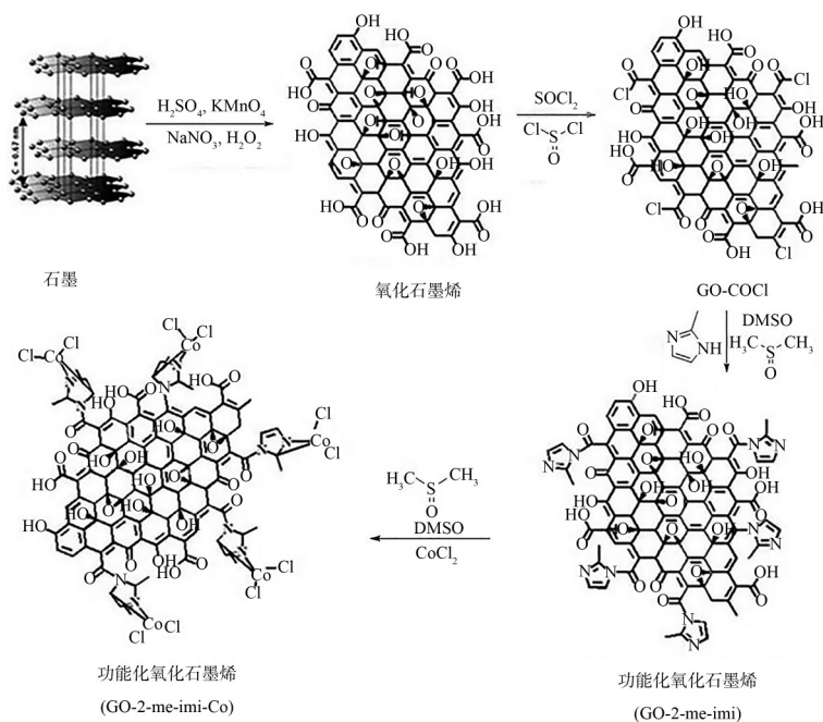
图5 合成GO-2-me-imi-Co的路线图 [15]
