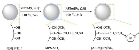
图10 [ARIm][Br]/SiO 2 颗粒合成示意图 [20]
